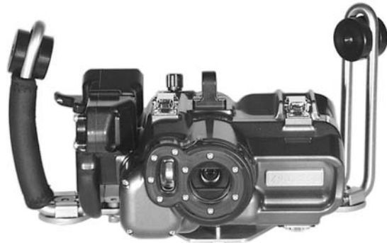
ビデオハウジング ZP-GS250 セット例
